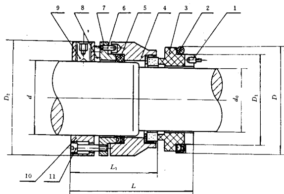
图 8 B105 型机械密封
