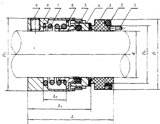
图 3 104 型机械密封
