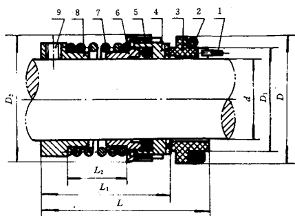
图 1 103 型机械密封
