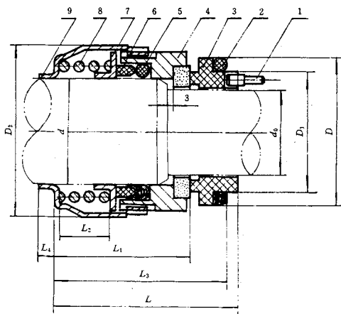
图 6 B104a 型机械密封
