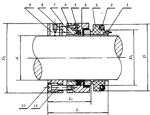
图 7 105 型机械密封
