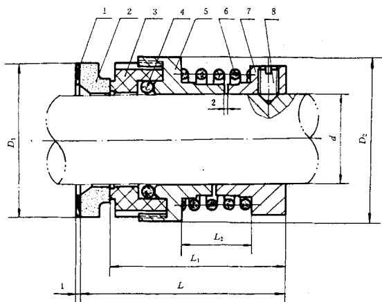
图 9 114 型机械密封
