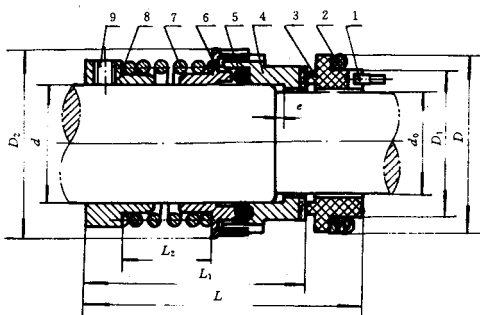
图 2 B103 型机械密封
