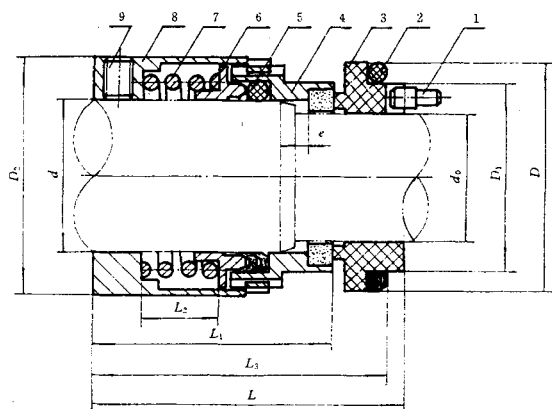
图 5 B104 型机械密封
