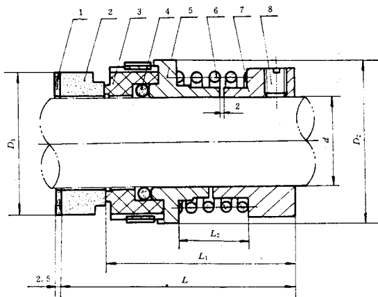
图 10 114a 型机械密封
