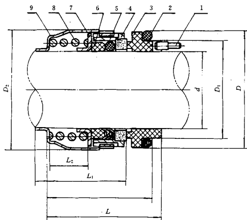
图 4 104a 型机械密封
